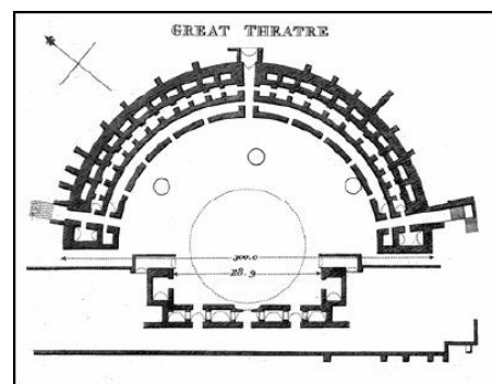
Κάτοψη του Θεάτρου της Νικόπολης. Σχέδιο του T.L. Donaldson, 1835
