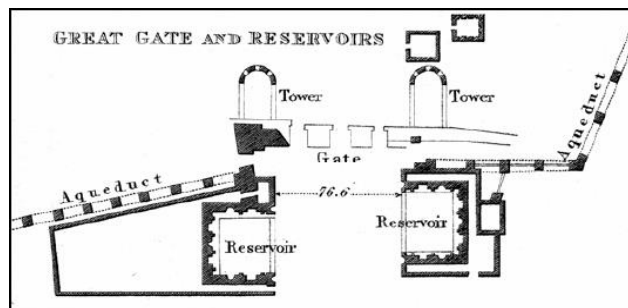
Κάτοψη των Νυμφαίων και της δυτικής πύλης της ρωμαϊκής Νικόπολης. Σχέδιο του T.L. Donaldson, 1835
